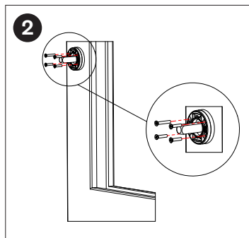
Fissarlo con le 4 viti Fix the mechanism with 4 screws
