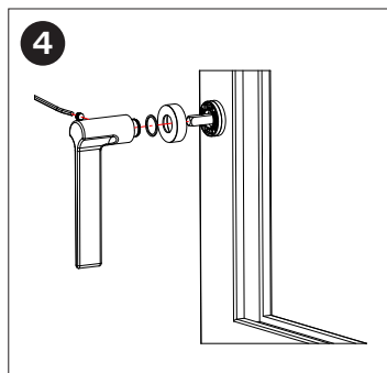
Inserire la rosetta, posizionare la maniglia e bloccarla con il grano Insert the rose, place the handle and lock it in position with the grub screw
