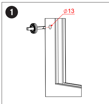
Inserire il meccanismo Insert the mechanism
