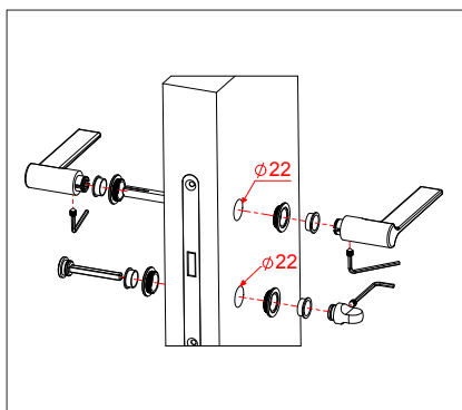
Con nottolino With turn & release
